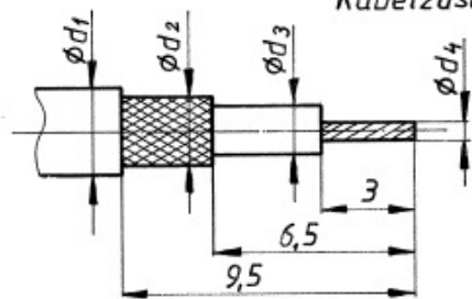
Kabelzuschnitt
